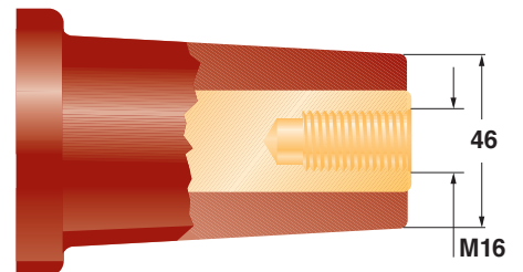
Бушинг типа С
